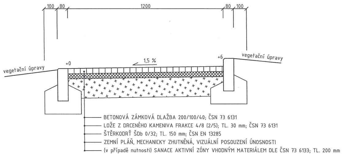
Obrázek 4 - Schématický vzorový řez
