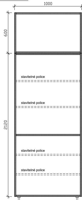
řez 2 - 2
