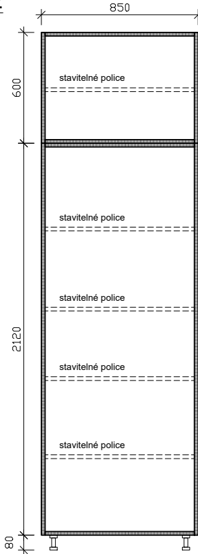
řez 2 - 2
