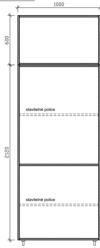
řez 2 - 2
