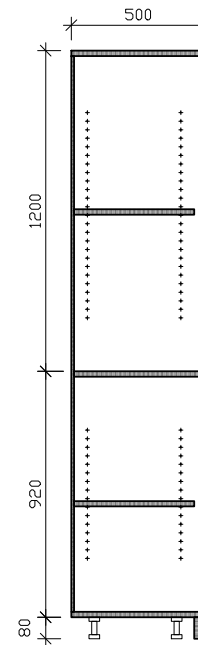
řez 3 - 3
