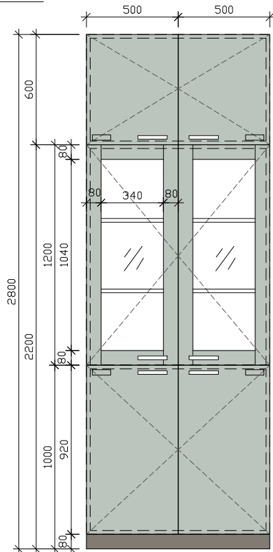
pohled 1 - 1
