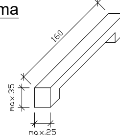
řez 3 - 3
