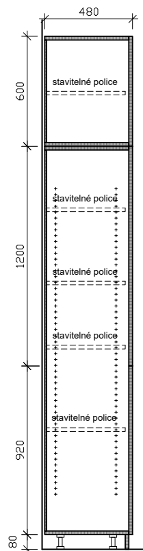
řez 3 - 3
