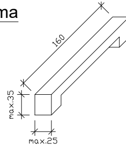
řez 3 - 3
