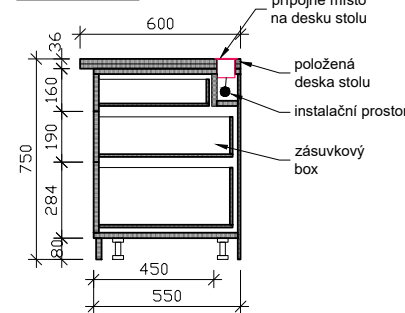
řez 2 - 2
