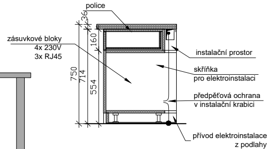
řez 2 - 2
