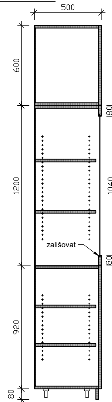
řez 3 - 3
