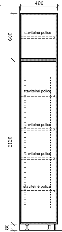
řez 3 - 3
