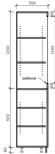
řez 3 - 3
