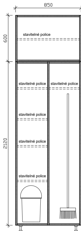
řez 2 - 2
