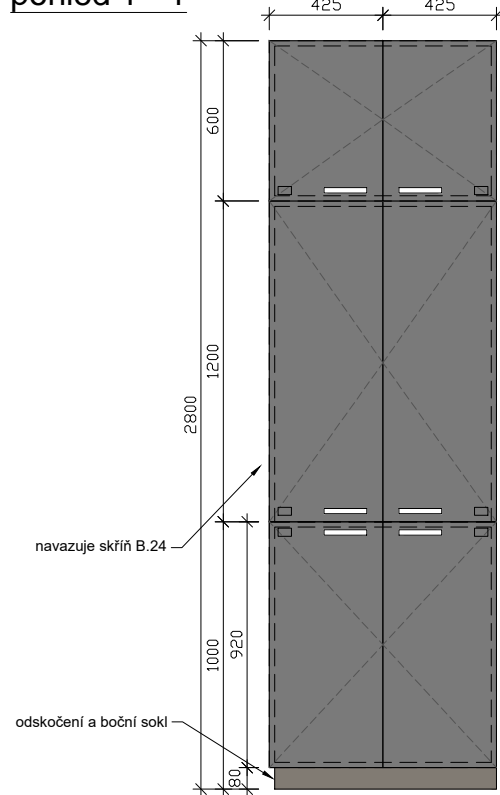
pohled 1 - 1
