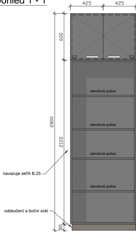
pohled 1 - 1
