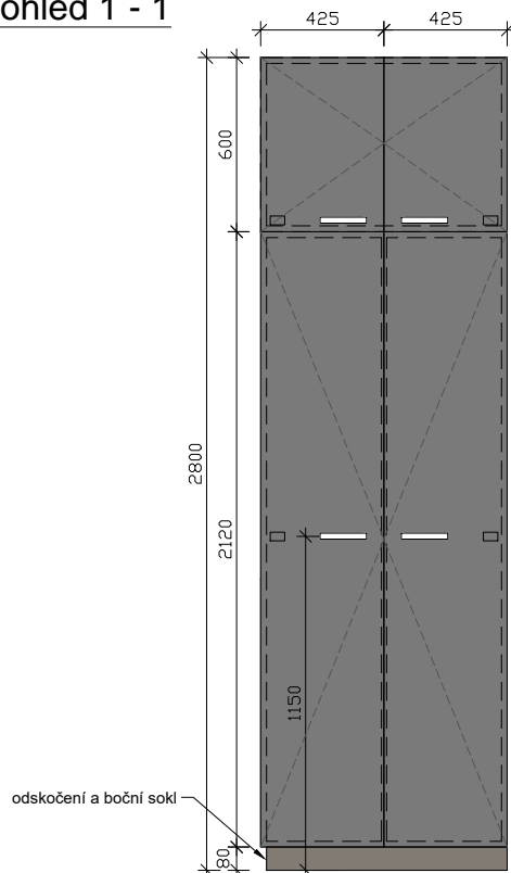
pohled 1 - 1
