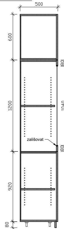
řez 3 - 3
